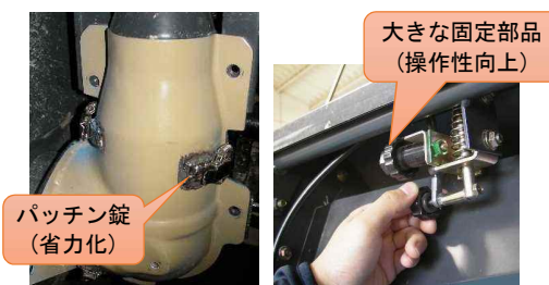
図3 開閉簡便な掃除口の例
