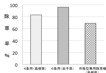
図3 開発機の除草効果 島根県での試験は2回除草（移植後5日、15日） 岩手県での試験は3回除草（移植後9日、16日、21日） 除草時期6月、試験面積10a、作業速度約1.1~1.2m/s 市販型乗用除草機は作業速度約0.6m/s
