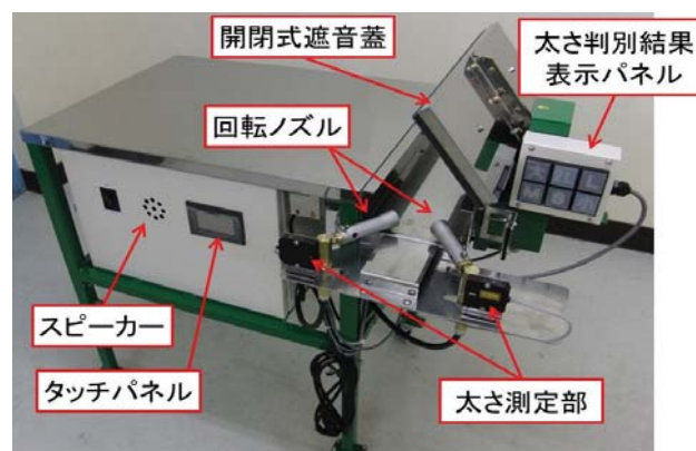
図2 試作3号機
