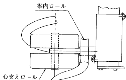
図2 心支えロールと案内ロール
