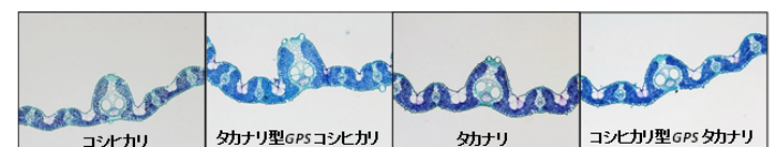
図 3. 各品種・系統の葉身断面
