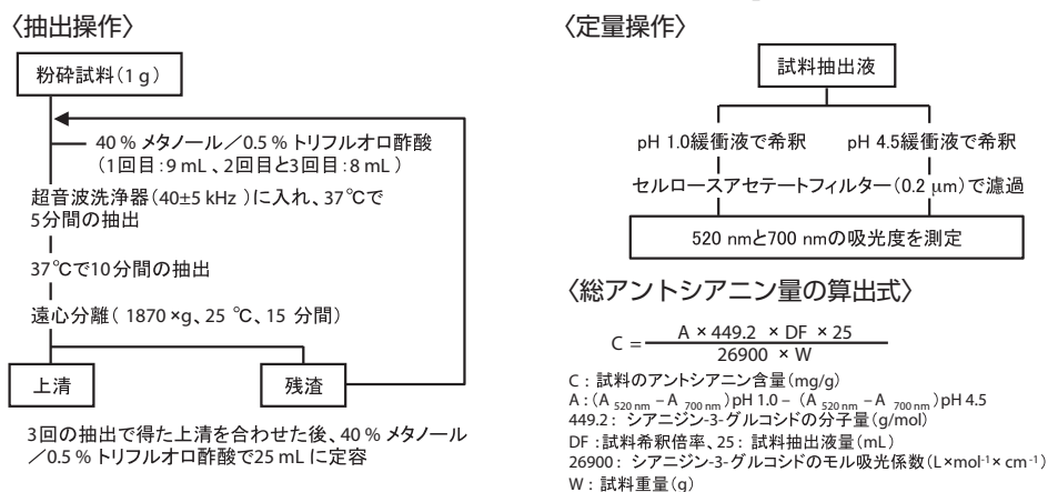
図 1 紫黒米と黒大豆中の pH differential 法による総アントシアニンの測定法の概要
