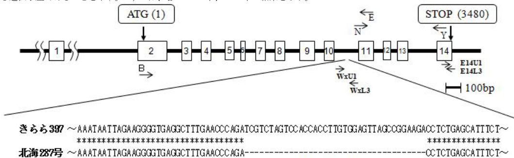
図2. ワキシー ( wx ) 遺伝子の構造と解析に用いたプライマーの位置
