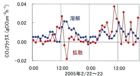
図3 単位時間中に積雪層から出て行く二酸化炭素量の比較。赤線(拡散)は図2の赤矢印、青線(溶解)は青矢印に相当する。マイナスの値は、大気から積雪層への吸収を示す。
