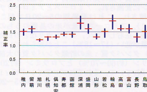
図3 雪について各地点の降水量補正率（補正後／観測値）。バーは風速の見積もりによる幅を、中央は平均値を示す。
