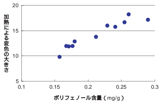
図 プロアントシアニジン系統大麦粉のポリフェノール含量と加熱後の変色の大きさとの関係 加熱後の変色が著しいものほど数字が大きくなる。
