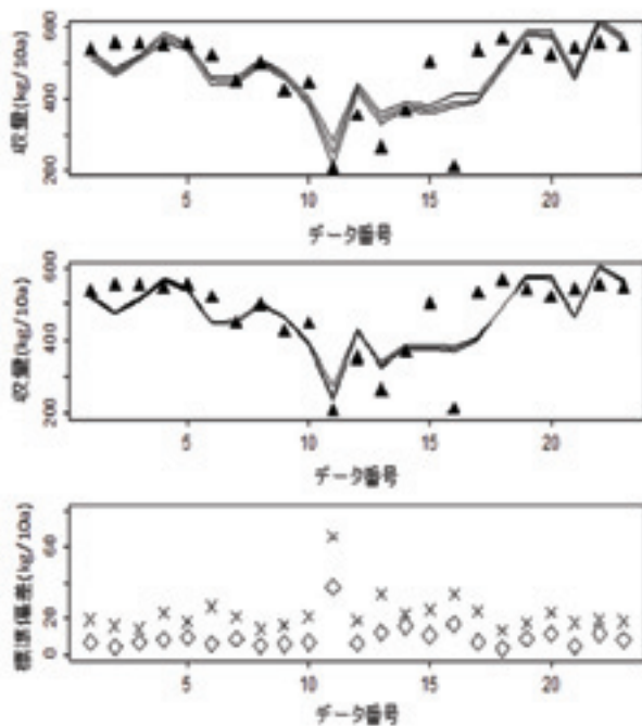
図1 従来の回帰(▲がデータ、3本線は、上から、信頼区間の上限、推定値、信頼区間の下限)(上)、重み付きの回帰(中)、推定値の標準偏差(xが重みなし、◇が重み付き)(下)
