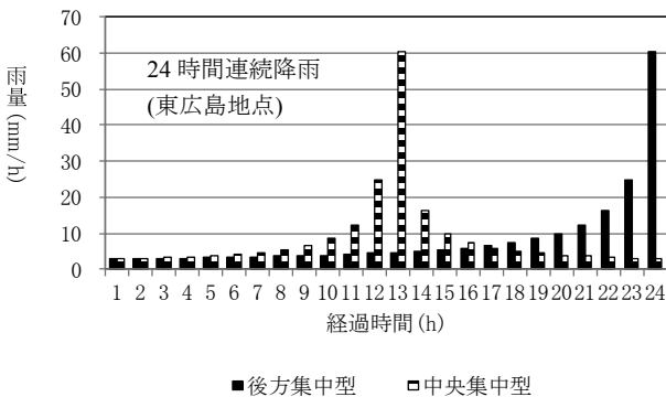
Fig.3-8 現在降雨のハイエトグラフの例(確率降雨30年) Example of the hyetograph of the present rain
