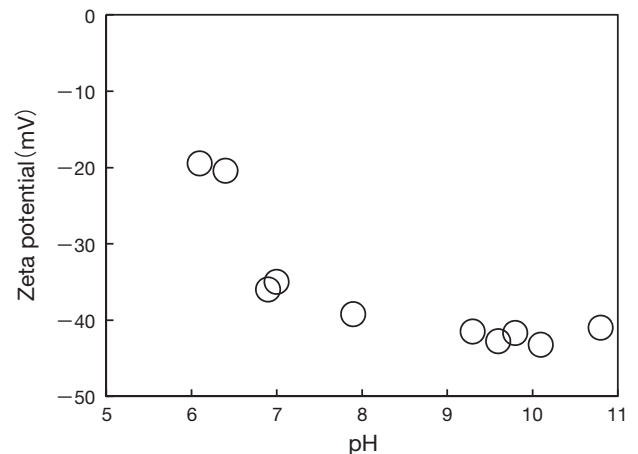
図2 土壌懸濁液pHとゼータポテンシャルの関係
