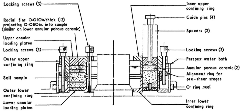
Fig.4 せん断箱の詳細 (Bishop 原図)
