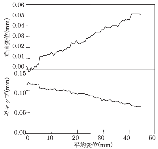
Fig.23 垂直変位及びギャップ (プレカット試料) Vertical displacement and gap (pre-cut sample)
