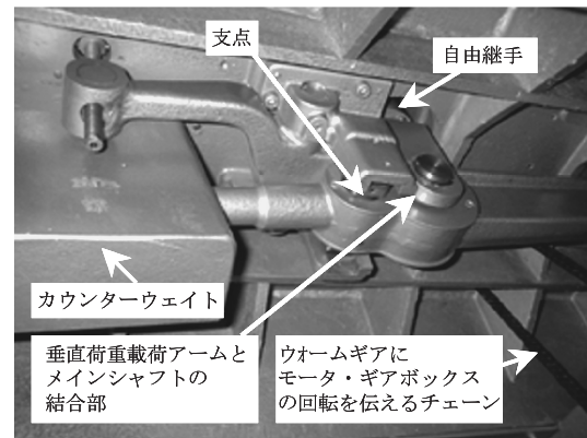
Fig.8 メインシャフト下方の自由継手
