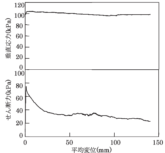
Fig.24 応力-変位関係 (過圧密試料)
