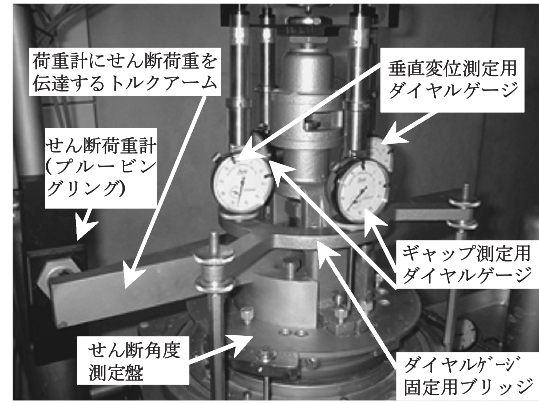
Fig.12 トルクアームで伝達されるせん断荷重
