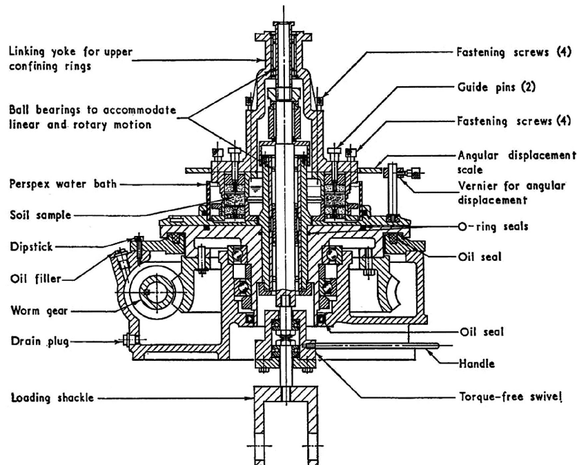
Fig.9 せん断上箱とリンク機構 (Bishop ら原図)
