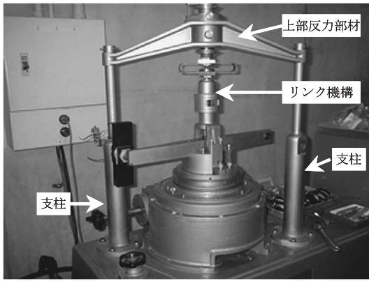
Fig.10 上部反力部材に結合されたリンク機構
