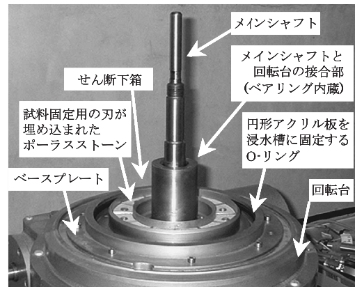
Fig.3 回転台に取付けられたベースプレート
