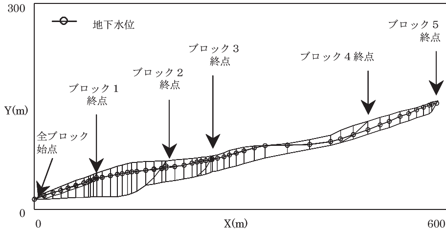
Fig.38 安定解析断面
