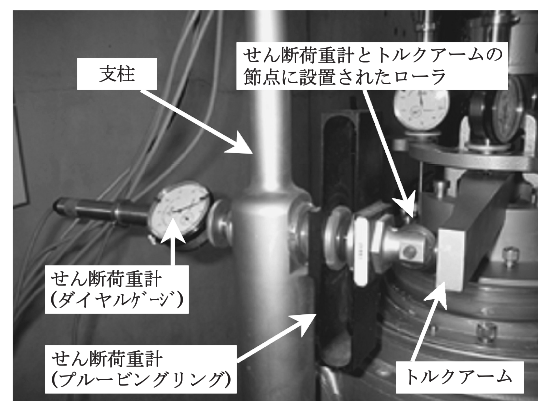
Fig.13 せん断荷重測定部
