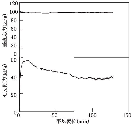
Fig.27 応力-変位関係 (正規圧密試料)
