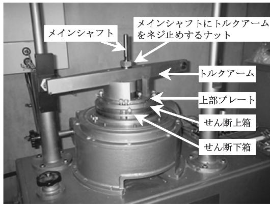
Fig.7 トルクアームで伝達される垂直荷重
