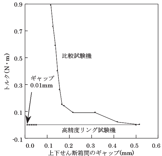
Fig.15 ブランクテストにおけるトルクとギャップの関係 Relationships between torque and gap in blank test
