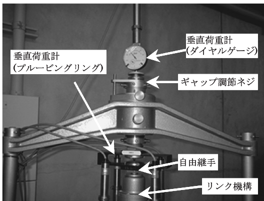
Fig.11 垂直荷重測定部
