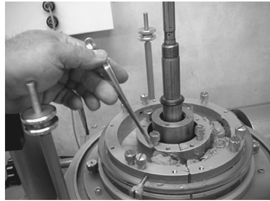
Fig.16 せん断箱へのスラリー試料充填
