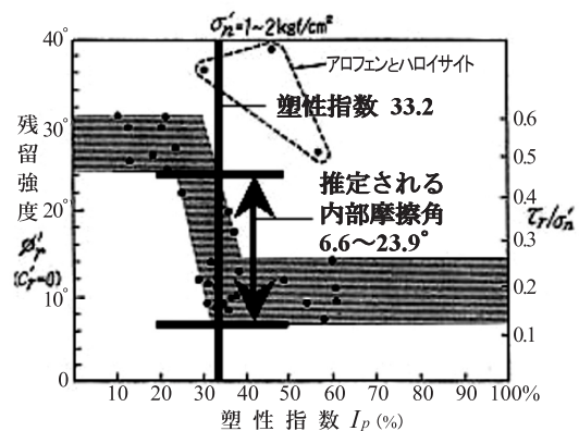
Fig.36 塑性指数と残留強度の関係
