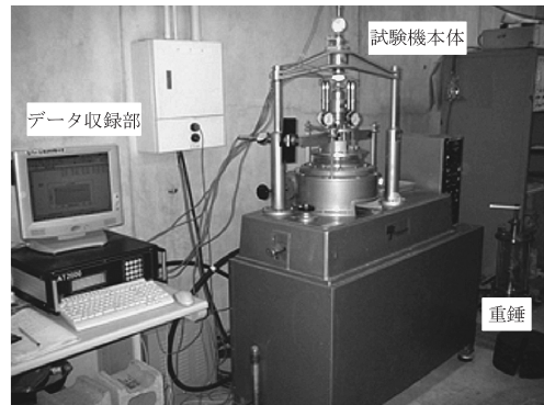
Fig.2 リングせん断試験機全景
