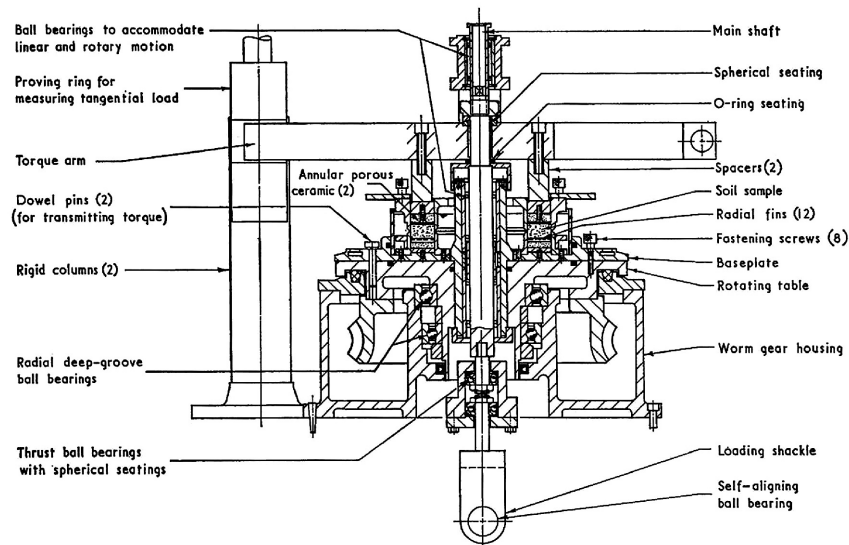
Fig.5 荷重伝達機構 (Bishop 原図)
