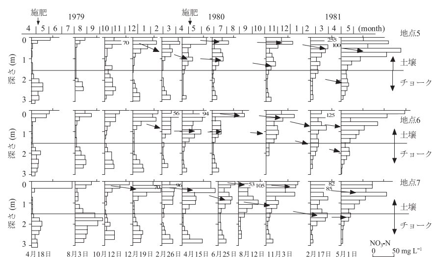
Fig.13 1979年から1981年の麦畑下のチョーク不飽和帯における硝酸性窒素濃度 (Wellings, 1984b)
