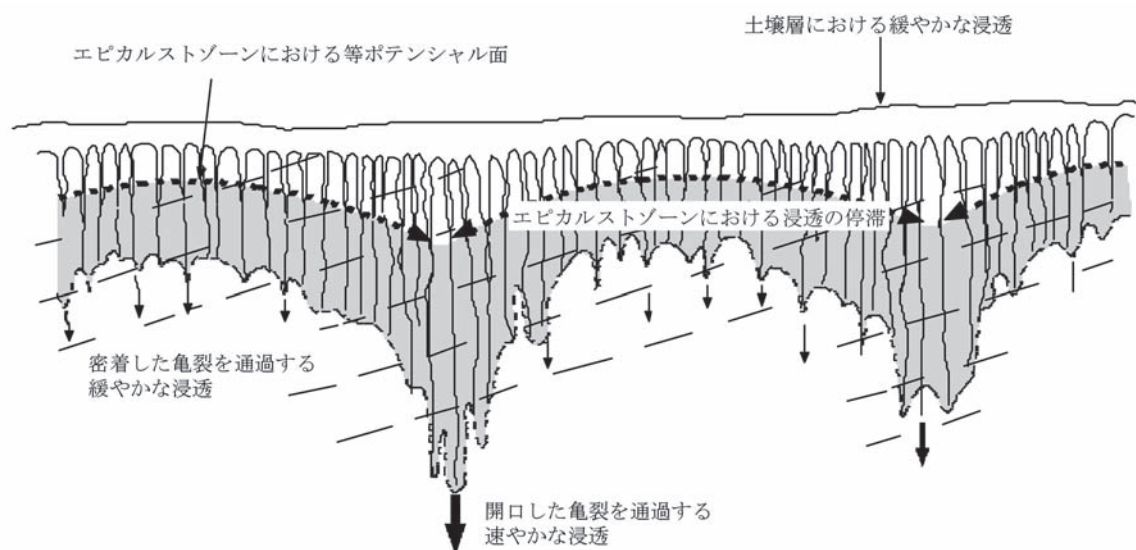
Fig.1 エピカルストゾーンにおける浸透水の貯留と高透水部への水平流動（Williams, 1983）
