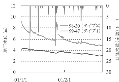
Fig.9 沖縄本島南部における地下水位変動の類別 (吉本ら, 2007)
