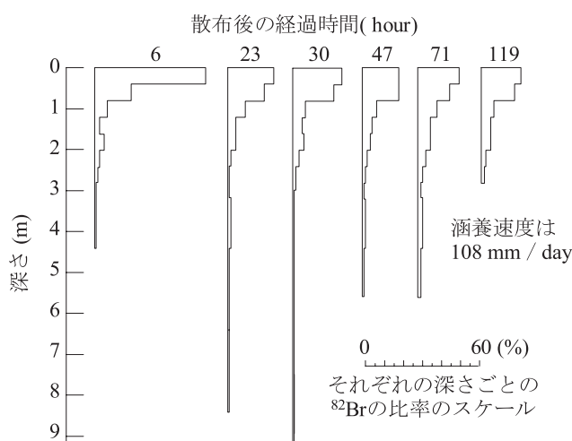
Fig.11 イギリスのチョーク帯水層における ^{82}\text{Br} トレーサの鉛直分布 (Black and Kipp, 1983)
