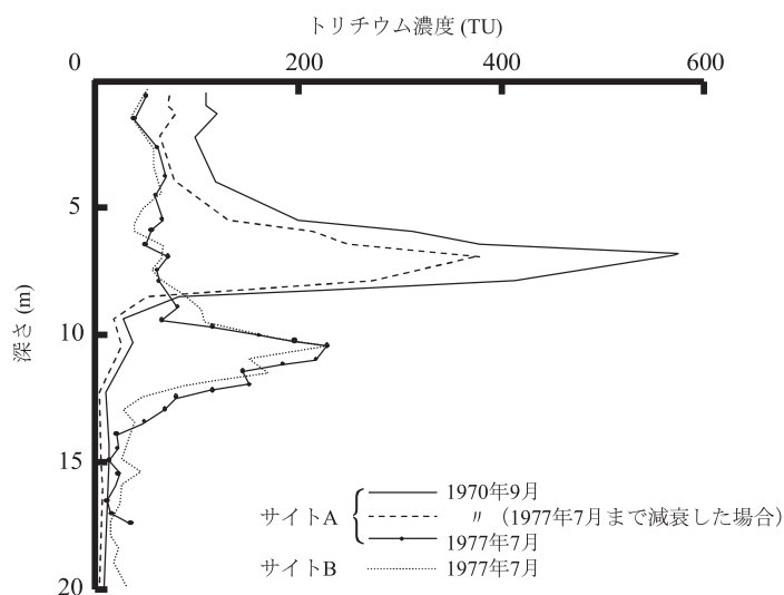
Fig.10 イギリス南東部のチョーク帯水層におけるトリチウムの鉛直分布 (Foster and Smith-Carington, 1980)
