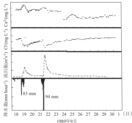
Fig.8 秋吉台・秋芳洞の地下河川における流出量と \text{Ca}^{2+} 、 \text{Cl}^- 濃度の変化（吉村・井倉, 2000）
