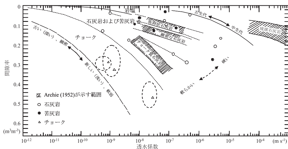
Fig.5 炭酸塩岩の間隙率と透水係数の関係（小鯛, 1984を一部改変）
