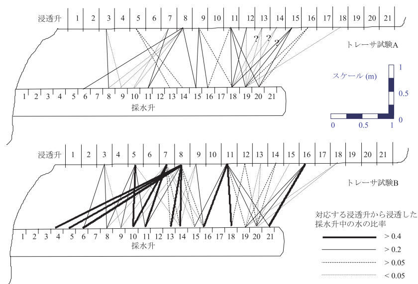
Fig.12 イスラエル・北ネゲヴ砂漠での浸透試験における不飽和浸透流の到達経路 (Dahan et al., 1999)
