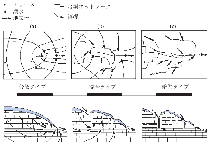
Fig.7 カルスト地形の発達と地下水流動の変化 (Quinlan and Ewers, 1985) Development of karst terranes and change in groundwater flow
