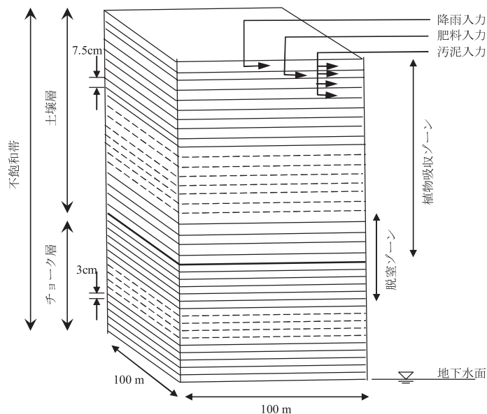
Fig.16 イギリスのチョーク帯水層に適用した1次元窒素溶脱モデル (IMPACT) の概念図 (Andrews et al., 1997a)
