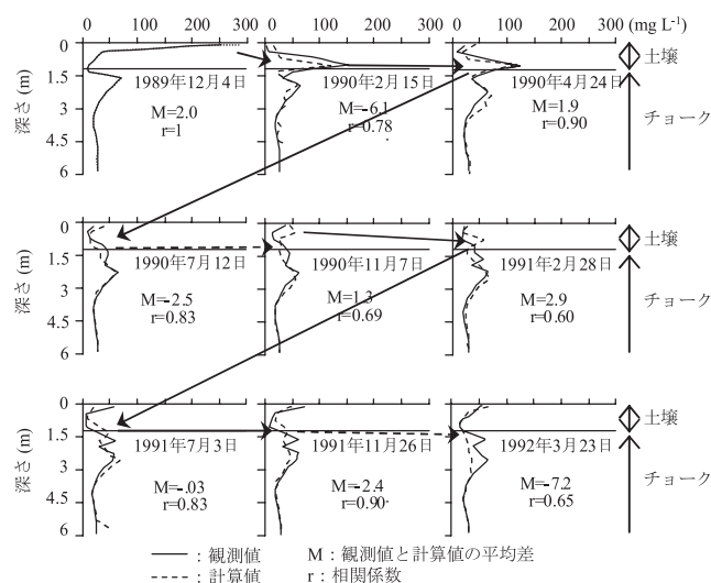
Fig.14 農場における硝酸塩濃度の鉛直分布 (Andrews et al., 1997b)
