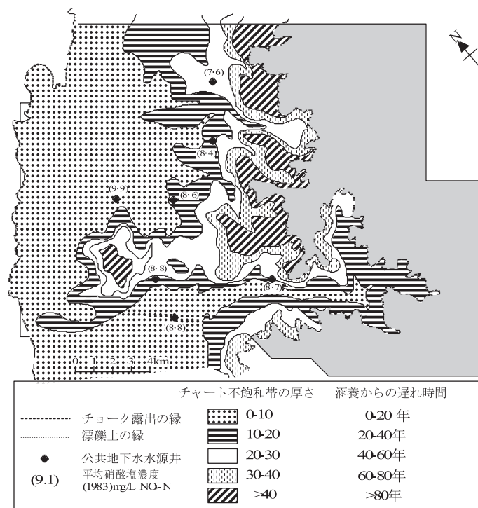
Fig.15 イギリス・ケンブリッジ周辺における不飽和帯水層の厚さ分布および窒素負荷の遅れ時間 (Carey and Lloyd, 1985)
