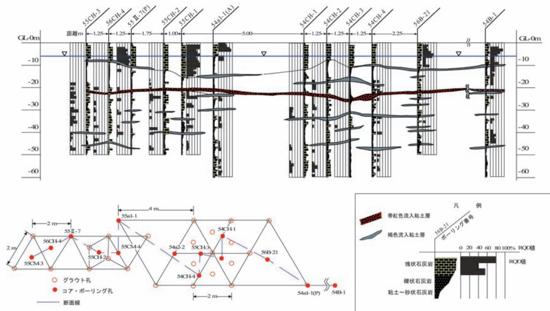
Fig.3 グラウト試験地における流入粘土の分布状況 (今泉ら, 2002) Geological section of grouting test field
