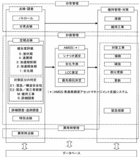
Fig.18 青森県の橋梁維持管理体系 (青森県土整備部道路課, 2004)
