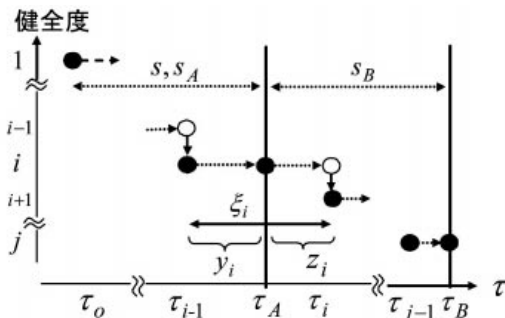
注) 初期時刻 \tau_0 から時間 s_A が経過した時刻 \tau (図中では \tau_A ) に健全度 i が観測される。ここでは、2つの検査時刻 \tau_A と \tau_B に着目する ( s_A = \tau_A - \tau_0 , s_B = \tau_B - \tau_A )。その場合、時刻 \tau_{i-1} から時刻 \tau_A までの期間長を y_i 、時刻 \tau_A から時刻 \tau_i までの期間長を z_i と表し、健全度 i の寿命を \xi_i = y_i + z_i と表す。
