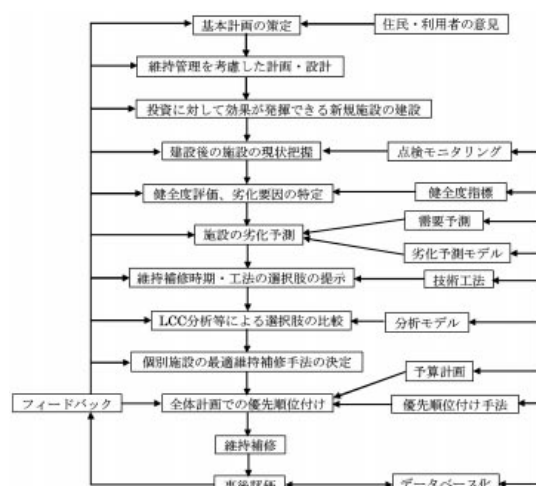
Fig.3 新規の農業水利施設の狭義のアセットマネジメントシステム Narrow Asset Management System for New Irrigation Infrastructure
