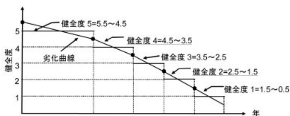
Fig.20 劣化曲線 (Matsumura et al., (2006) より作成) Deterioration Curve
