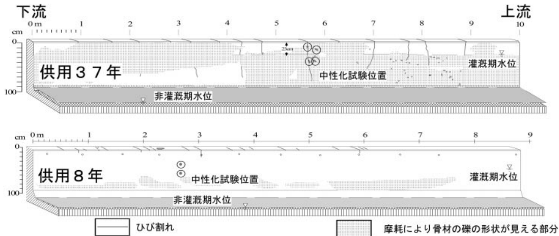
Fig.23 N地区の鉄筋コンクリート水路のびひ割れの分布状況
