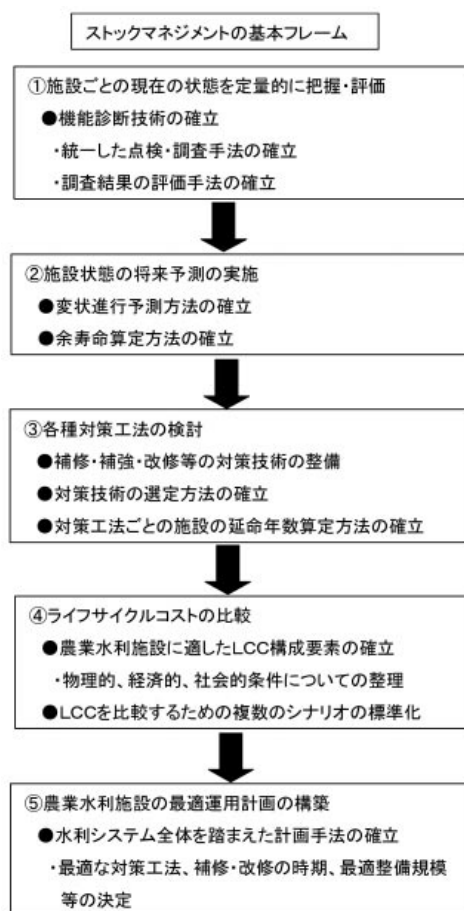
Ap-Fig.7 農業水利施設のストックマネジメントの基本フレーム (森, 2005)
