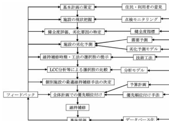
Fig.2 既存の農業水利施設を対象とした狭義のアセットマネジメントシステム Narrow Asset Management System for Existing Irrigation Infrastructure
