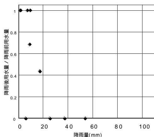
Fig.6 降雨量とそれによる用水流量減少(登熟期) Irrigation discharge decrease and rainfall (Ripening stage)
