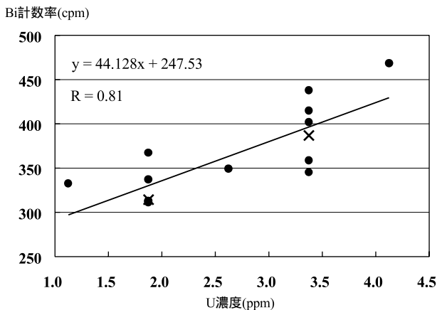
Fig.10 ^{214}\text{Bi} の線計数率とU濃度の比較
