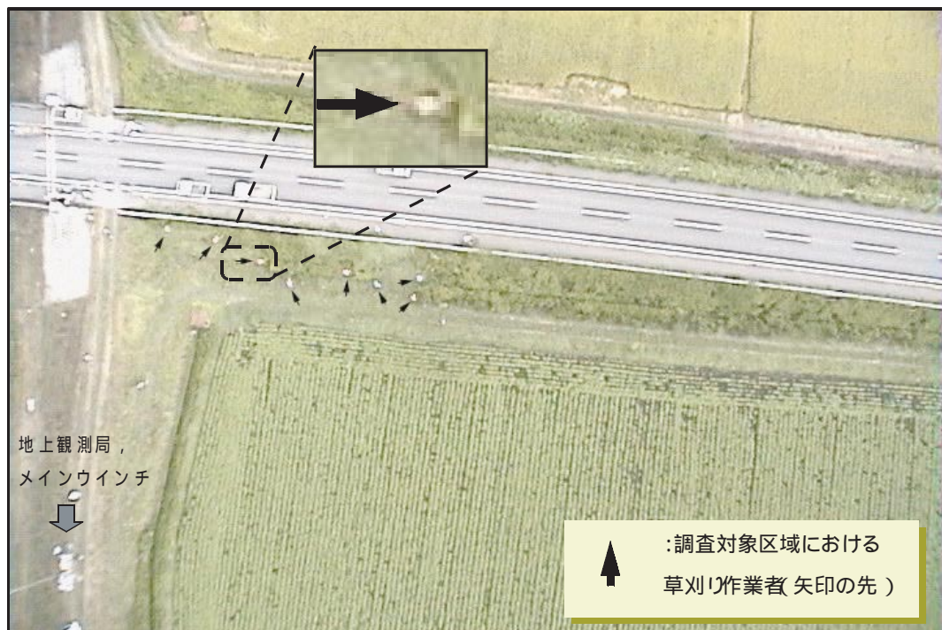
Fig.7 本システムによる草刈り作業状況を示す静止画像（幾何補正前： 720 \times 480 ピクセル）
