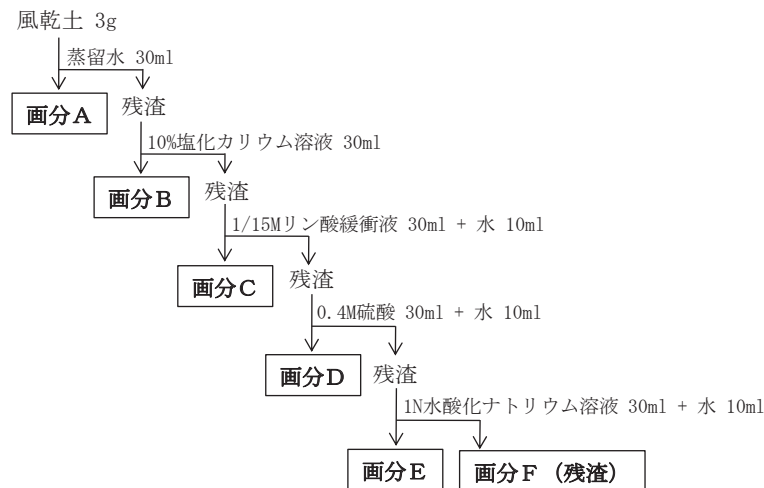
図2 現地試験にてサンプリングした土壤の窒素の逐次抽出手順.
