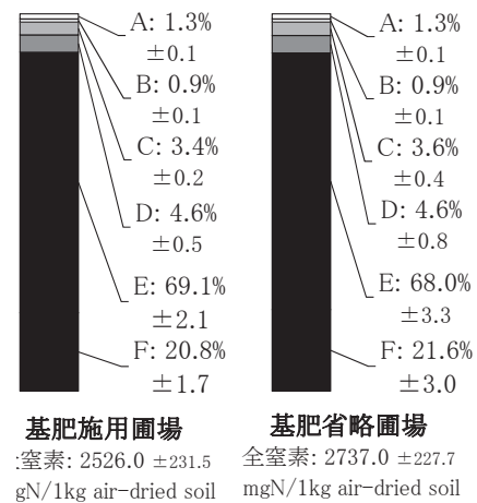
図4 現地試験におけるダイズ栽培後の土壤の窒素構成比。
