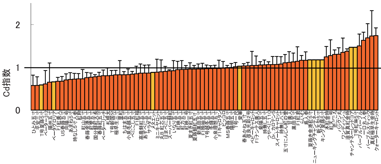
図1 ニンジン類84品種のCd濃度順位
