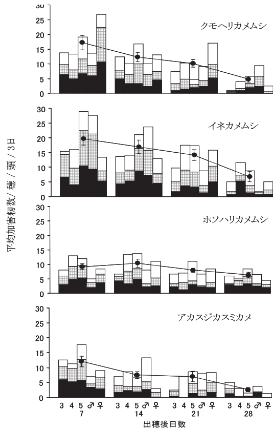
図30 カメムシ種、カメムシの発育段階、出穂後日数別の総加害羽数の平均値および穂内区分ごとの加害羽数の平均値。
