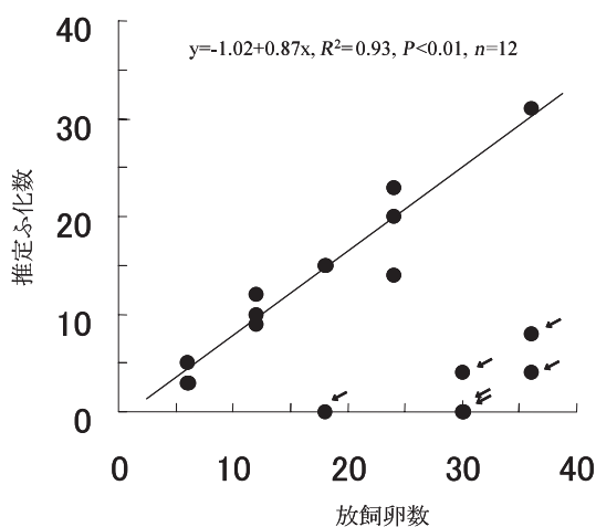
図10 水田内に設置した網枠内における放飼卵数と推定ふ化数との関係
