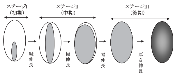
図32 籾の登熟段階の3つの区分。
