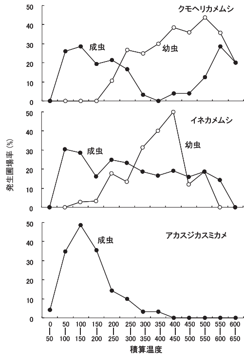
図36 クモヘリカメムシ、イネカメムシ、アカスジカメムシの発生圃場率の推移。
