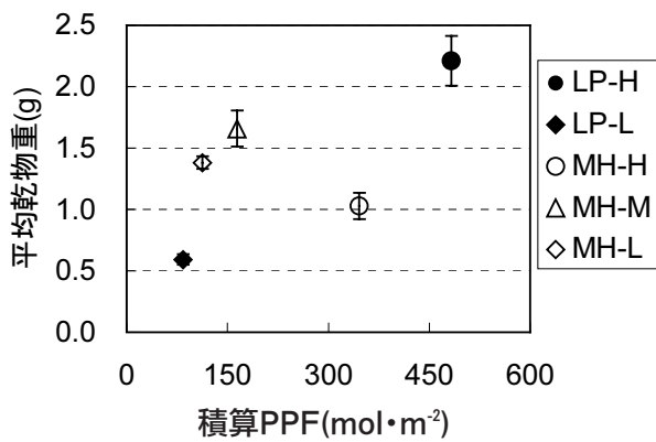
図-6 各処理区における積算光合成有効放射と乾物重との関係 エラーバーはstandard error(n=12)を示す。
