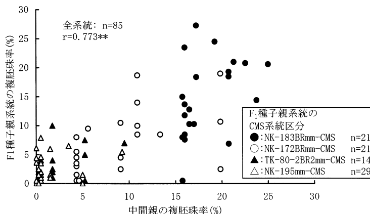
第24図 CMS系統区分による中間親の値とF 1 種子親系統の複胚珠率との関係(2001) **は1%水準で有意。
