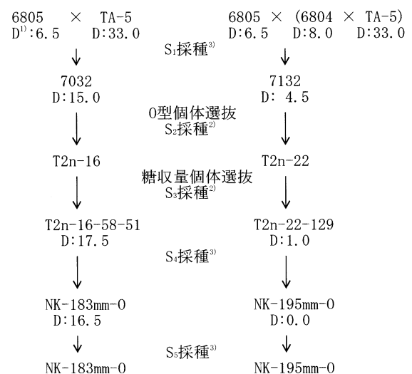
第22図 供試O型系統の育成系譜と複胚珠性
