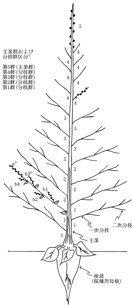
第16図 採種テンサイの主茎ならびに 分枝の区分模式図
