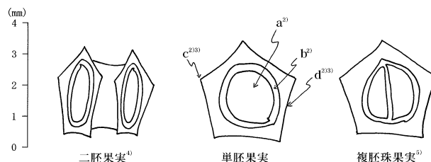
第2図 テンサイ単胚果実の分類模式図 1)
