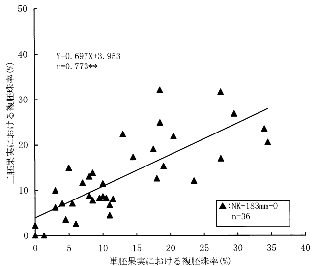
第21図 「NK-183mm-O」における個体単位の単胚果実と二胚果実における複胚珠率との関係 (1998)
