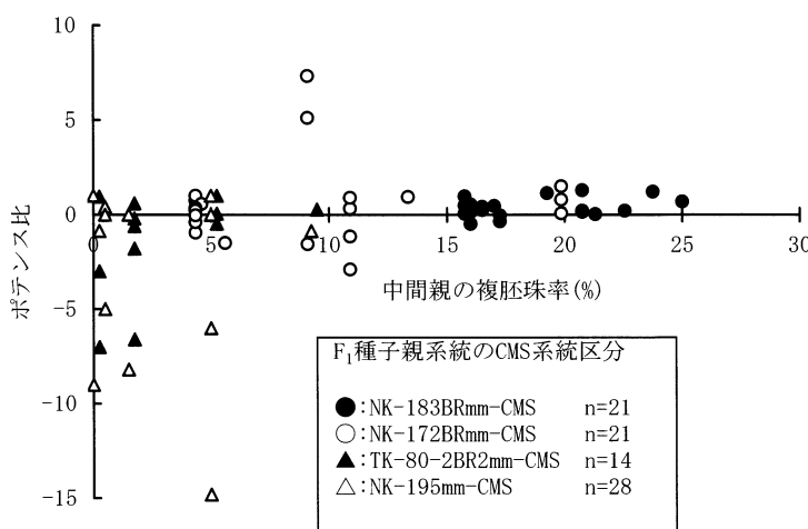
第25図 CMS系統区分によるF 1 種子親系統の複胚珠率に関する中間親の値とポテンス比との関係(2001)
