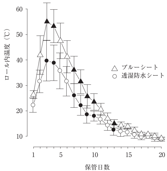
図3 ブルーシートおよび透湿防水シート被覆保管時における圧碎稲わらロール内温度の推移（平均値±標準偏差） 注. 黒印シンボルは有意差有（ P < 0.05 ）
